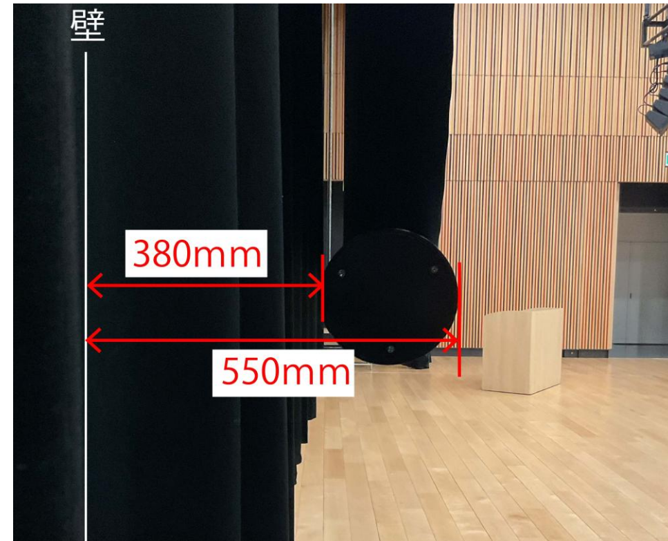
【壁からのスクリーンの寸法】
