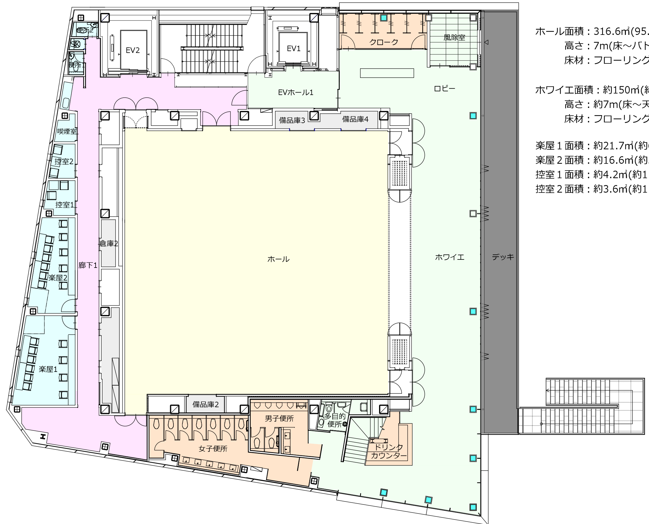
【2F平面図】
